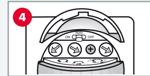
Handmatige schakelaar ON/OFF/AUTO De verlichting kan met behulp van de schuifschakelaar als volgt worden geschakeld: ON = permanent AAN OFF = permanent UIT AUTO = automatische modus, melder actief
