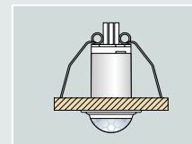
Med vedlagte fjederklemmer
