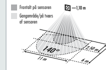
PD-C360i/6 mini, MD-C360i/6 mini
