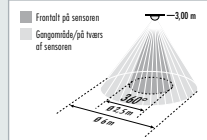
MD-C360i/6 mini
