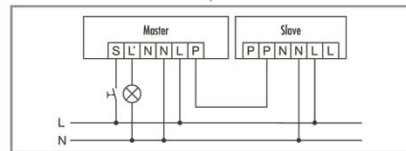
Master-slave-kobling: masterenheden styrer de tilsluttede forbrugssteder efter de indstillede parametre. Slaveenhederne udfører kun tilstedeværelsesdetektering og afgiver en impuls til masterenheden når de opdager bevægelse.
