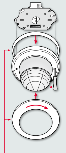
Inbouw IP 20 Inbouw/installatiedoos
