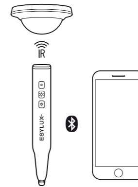
Standaardconfiguratie van alle op afstand bedienbare ESYLUX-producten met de ESY-App en de ESY-Pen als brug (IR)
